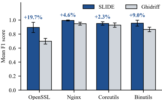
(a) Average F1 Score
