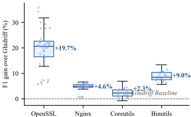
(b) Per-sample F1 Gain Distribution
